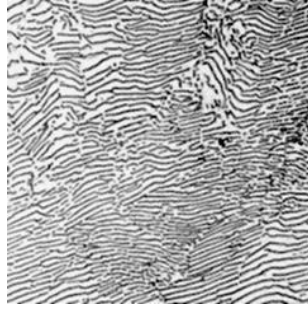
perlite
