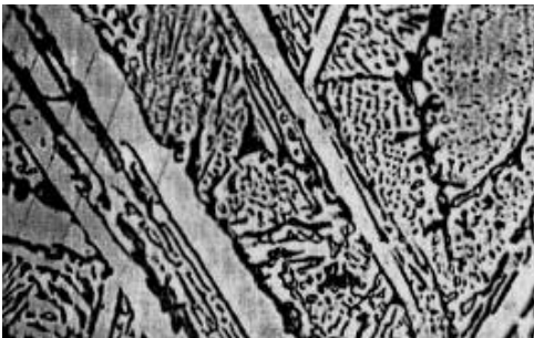
perlite + cementite II + ledeburite trasformata
