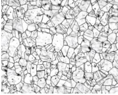
austenite
